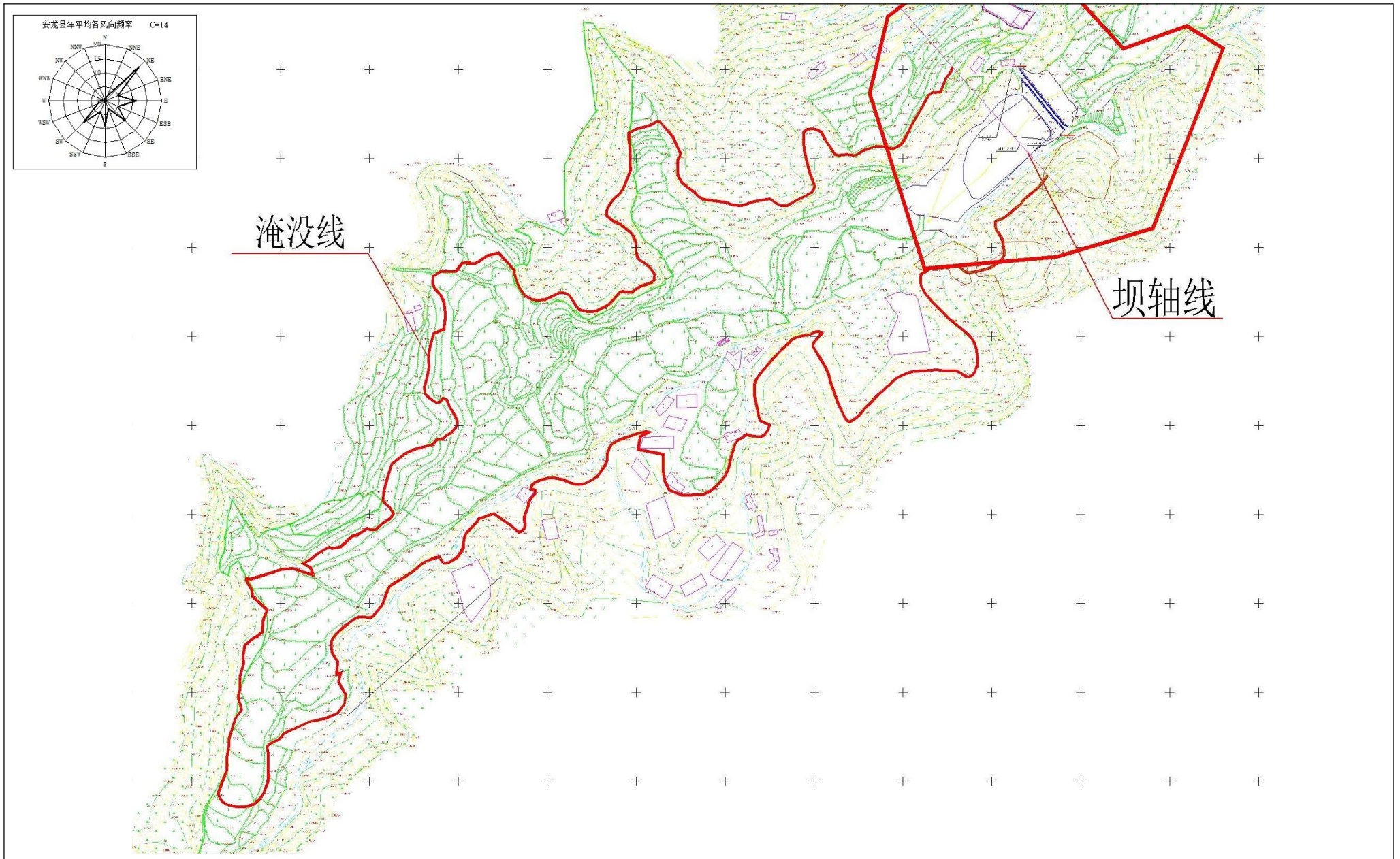
附图 3 安龙县龙洞水库淹没区占地范围图
